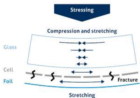
Glass-foil module
